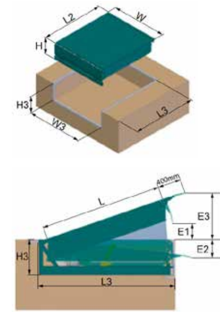
Estructura estándar para RH11, 2000L x 2500W x 600H (pit 2580 x 2040). 6t.
